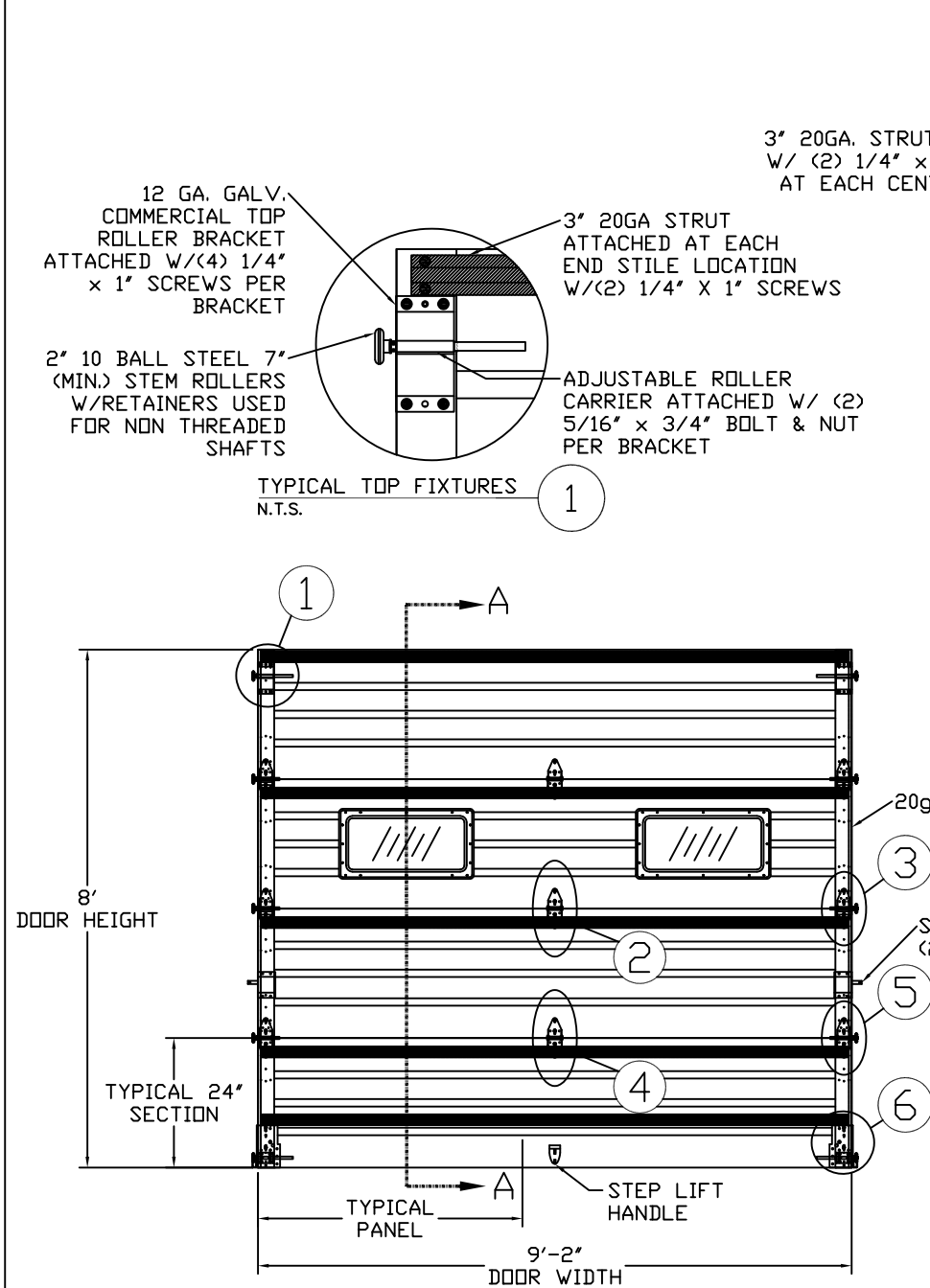
DOOR INTERIOR ELEVATION N.T.S.
