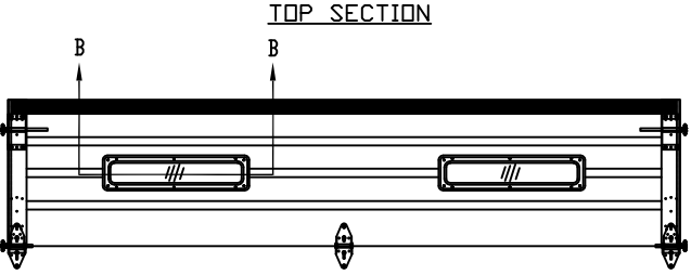
OPTIONAL GLAZED SECTION W/ 24" X 6" WINDOWS N.T.S.
