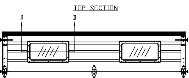
OPTIONAL GLAZED SECTION W/ 24" X 12" WINDOWS N.T.S.
