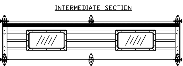
OPTIONAL GLAZED SECTION W/ 24" X 12" WINDOWS N.T.S.
