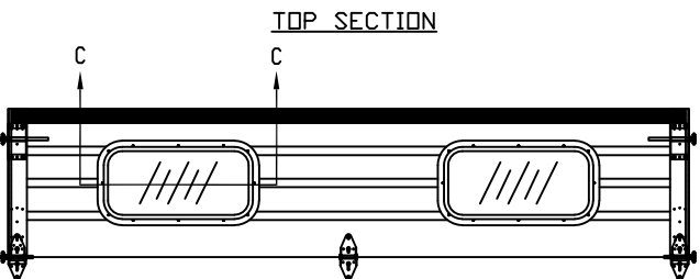
OPTIONAL GLAZED SECTION W/ 26" X 13" WINDOWS N.T.S.
